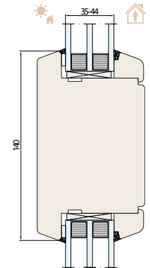
SYSTEM NATURO 80 szpros konstrukcyjny 140 mm
