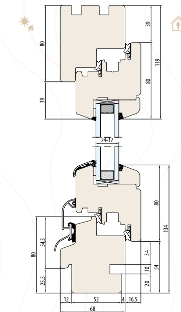
SYSTEM NATURO 68 podcięcie pod parapet wewnętrzne i zewnętrzne
