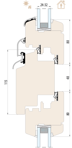
SYSTEM NATURO 68 ślemię 115 mm
