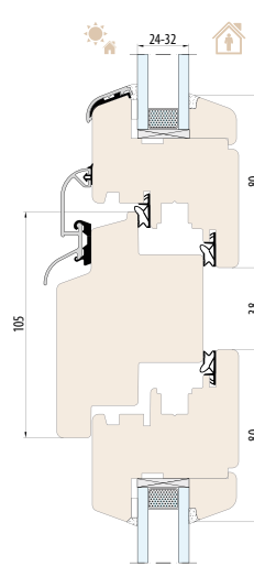
SYSTEM NATURO 68 ślemię 105 mm
