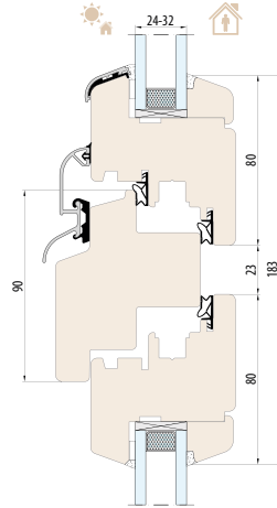
SYSTEM NATURO 68 ślemię 90 mm
