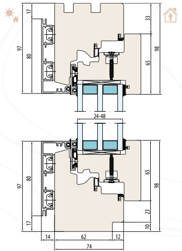
SYSTEM ESPERIA LIFE 74 ALU podcięcie pod parapet wewnętrzne
