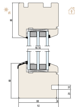
SYSTEM NATURO 92-Fix podcięcie pod parapet wewnętrzne
