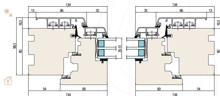
SYSTEM NATURO 80 ALU GEMINI CLASSIC PRZEKRÓJ POZIOMY B-B
