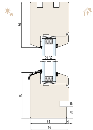
SYSTEM NATURO 68-Fix podcięcie pod parapet wewnętrzne
