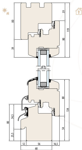
SYSTEM NATURO 68 podcięcie pod parapet zewnętrzne
