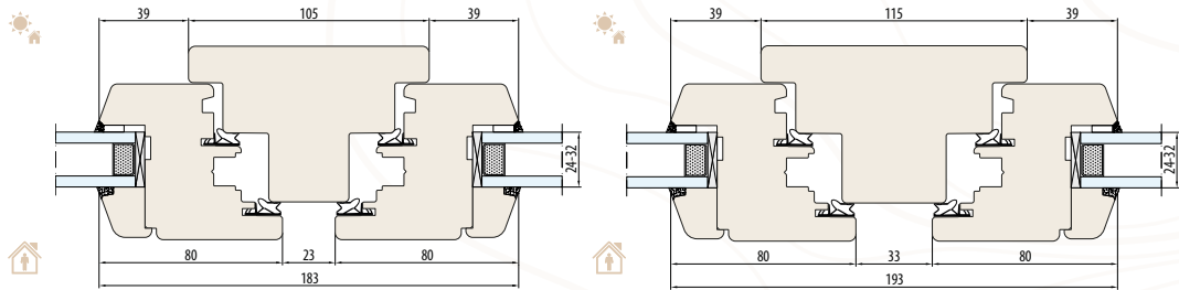
SYSTEM NATURO 68 słupek stały 105 mm (przekrój poziomy)
