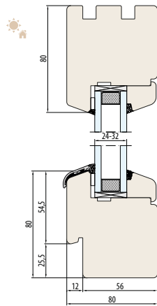
SYSTEM NATURO 68-Fix podcięcie pod parapet zewnętrzne
