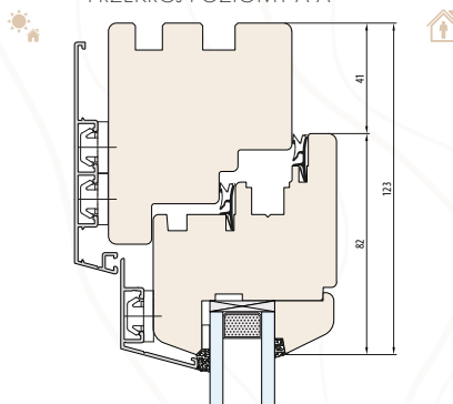
PRZEKRÓJ POZIOMY A-A
