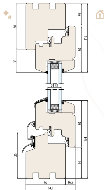
SYSTEM NATURO 68 bez podcięcia pod parapet
