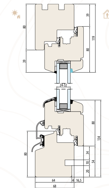
SYSTEM NATURO 68 podcięcie pod parapet wewnętrzne
