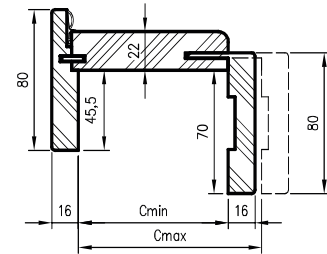
Cross-section of ościeżnicy
