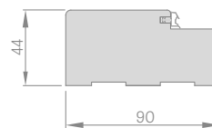
Fixed door frame
