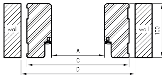
HORIZONTAL SECTION OP
