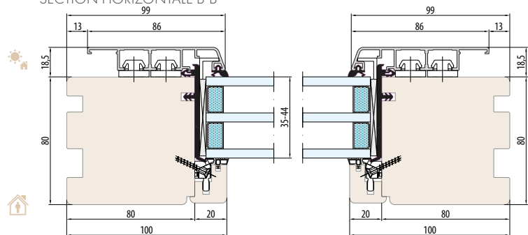
SYSTÈME NATURO 80 ALU-Fix GEMINI CLASSIC
