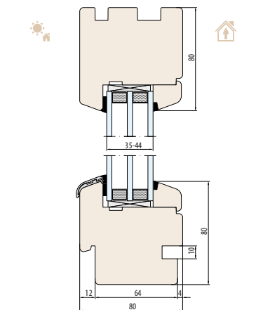
SYSTÈME NATURO 80-Fix découpe pour l'appui de fenêtre intérieur et extérieur
