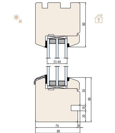
SYSTÈME NATURO 80-Fix découpe pour l'appui de fenêtre intérieur
